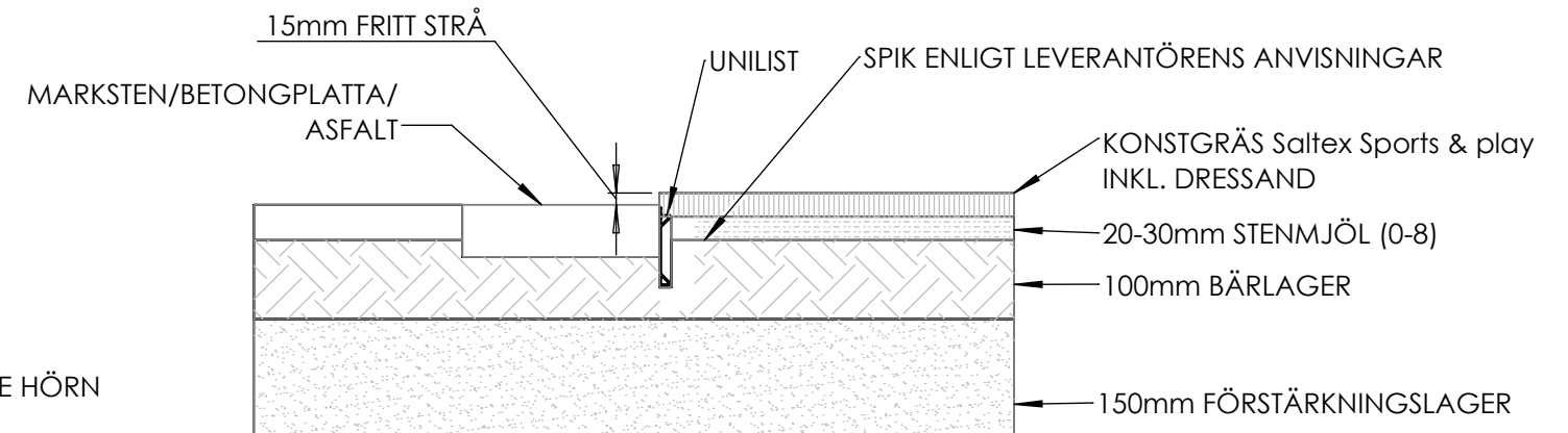
ANSLUTNING KONSTRÄS MOT HÄRDGJORDA YTOR MED UNILIST SKALA 1:10
