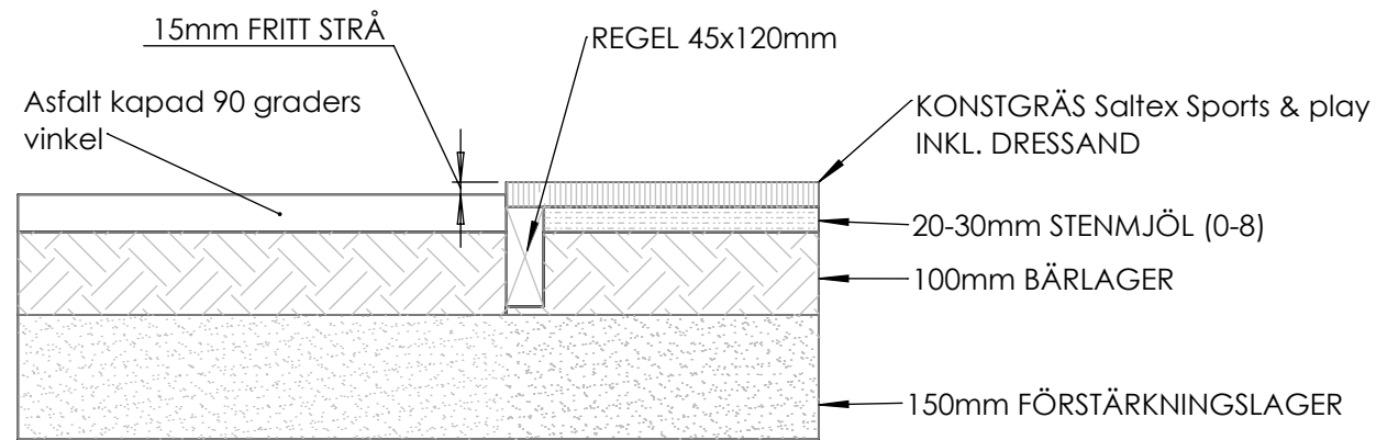
ANSLUTNING KONSTRÄS MOT ASFALT MED REGEL SKALA 1:10
