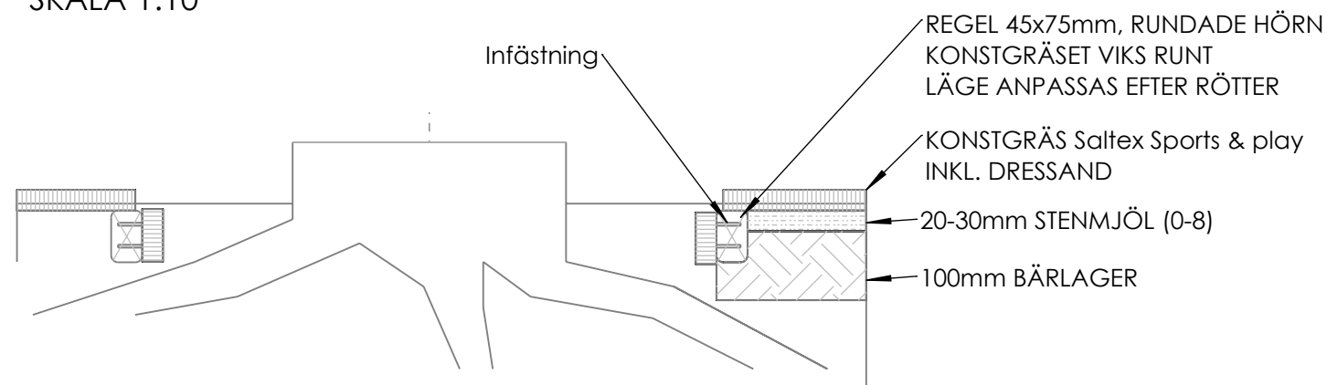
ANSLUTNING KONSTRÄS MOT TRÄD MED REGEL SKALA 1:10
