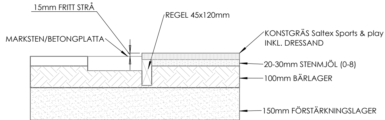
ANSLUTNING KONSTRÄS MOT KANTSTEN MED REGEL SKALA 1:10
