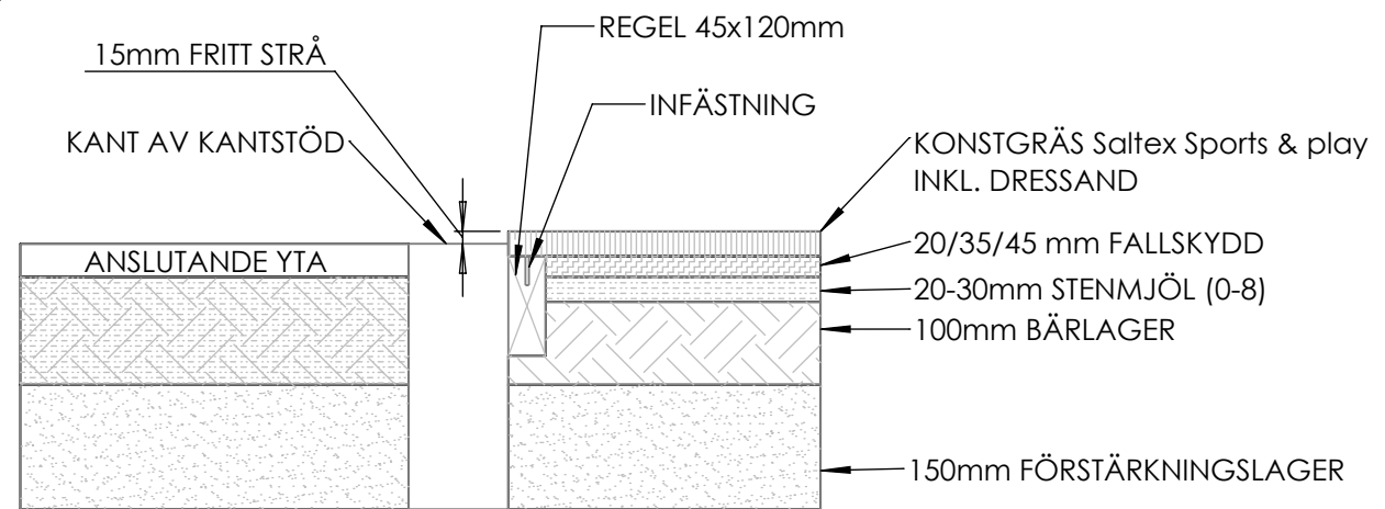
ANSLUTNING KONSTRÄS MED FALLSKYDD MOT KANTSTEN MED REGEL SKALA 1:10
