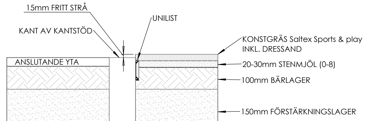
ANSLUTNING KONSTRÄS MOT KANTSTEN MED UNILIST SKALA 1:10
