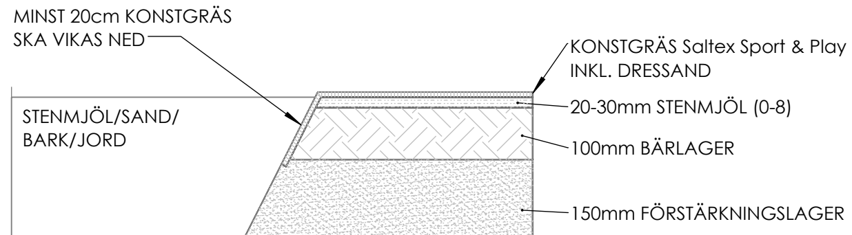
ANSLUTNING KONSTRÄS MOT LÖSA MATERIAL TYP STENMJÖL, SAND, BARK M.M. SKALA 1:10
