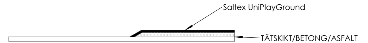
ANSLUTNING UniPlayGround PÅ BJÄKLÄG OCH ASFALT SKALA 1:10
