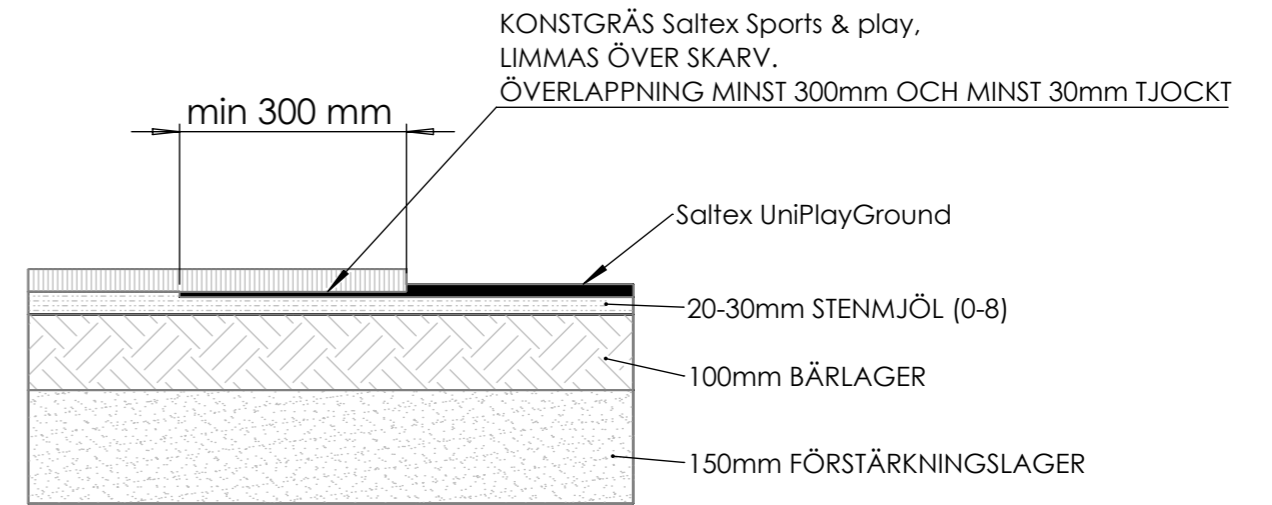
DOLD KANT UniPlayGround MOT KONSTGRÄS SKALA 1:10
