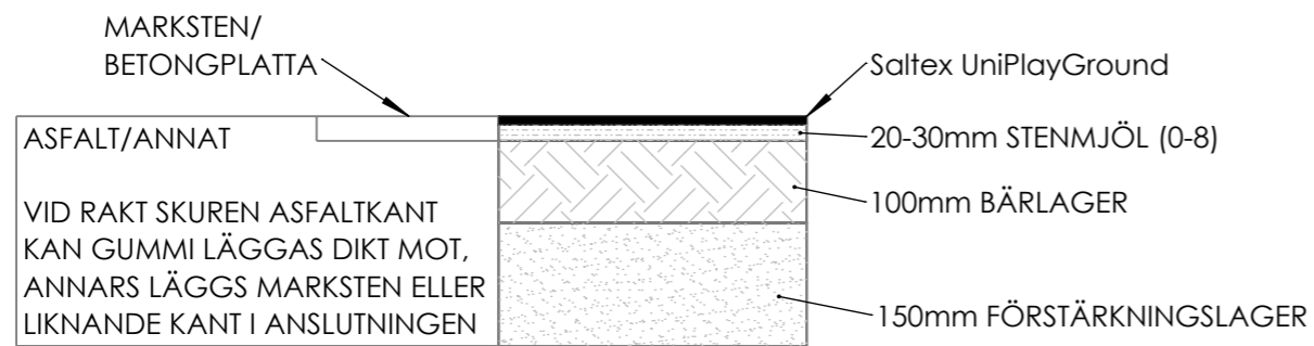
ANSLUTNING UniPlayGround MOT HÅRDGJORDA YTOR TYP ASFALT, BETONGMARKSTEN M.M. SKALA 1:10
