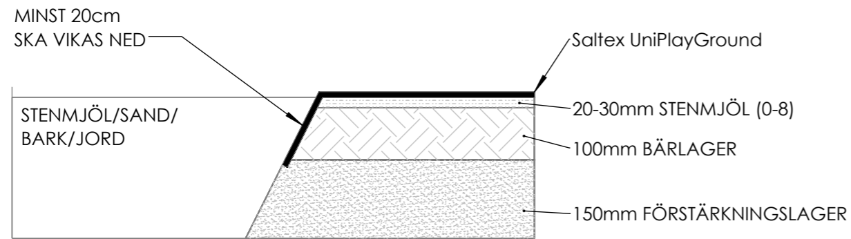
ANSLUTNING UniPlayGround MOT LÖSA MATERIAL TYP STENMJÖL, SAND, BARK M.M. SKALA 1:10
